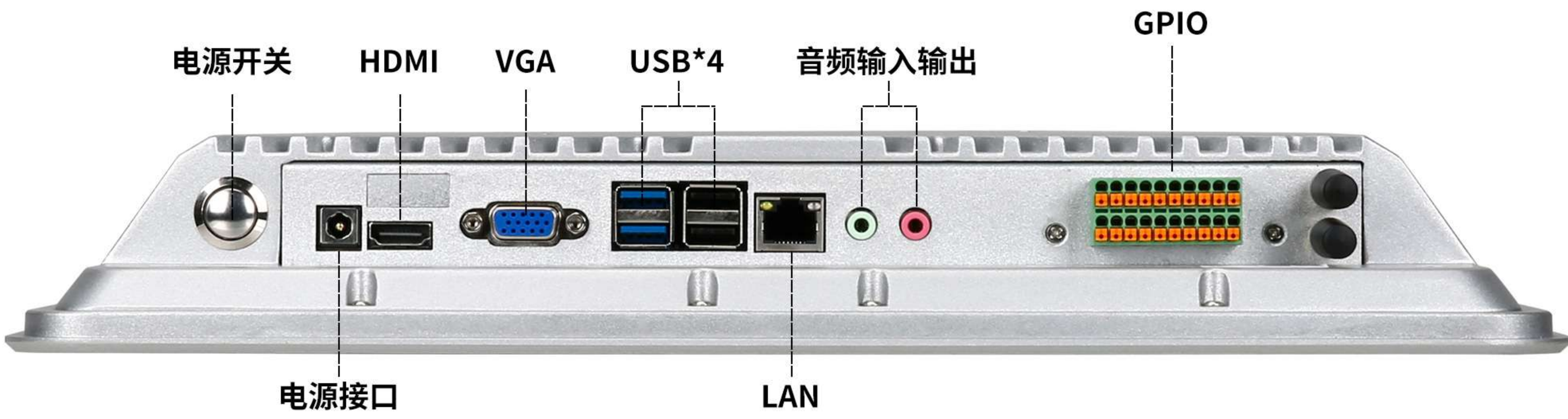
加装GPIO接口图
